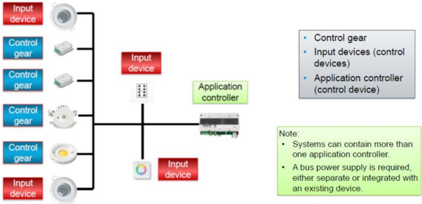
Figuur 5: Architectuur van een DALI-2 systeem (Bron DiiA)
